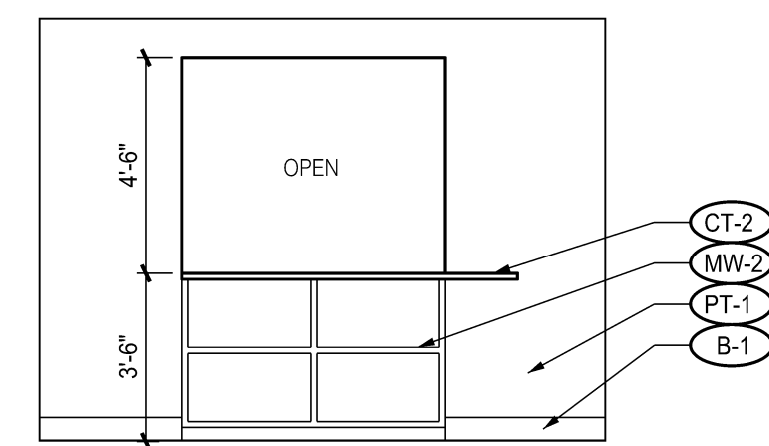
11 INTERIOR ELEVATION - CHECKIN A4.01 SCALE: 1/4" = 1'-0"
